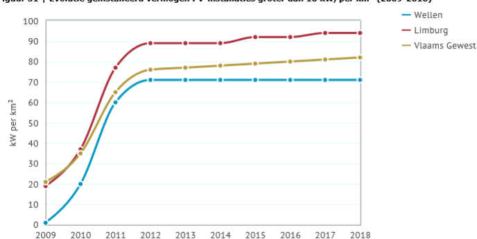
Figuur 51 | Evolutie geïnstalleerd vermogen PV-installaties groter dan 10 kW, per km 2 (2009-2018)
